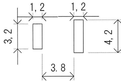
取付穴参考図
