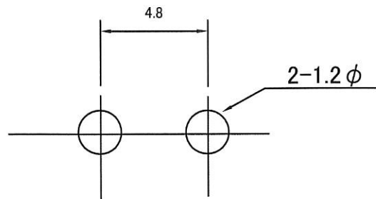
適合取付穴寸法図
