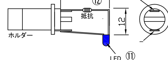
LEDランプ接続例
