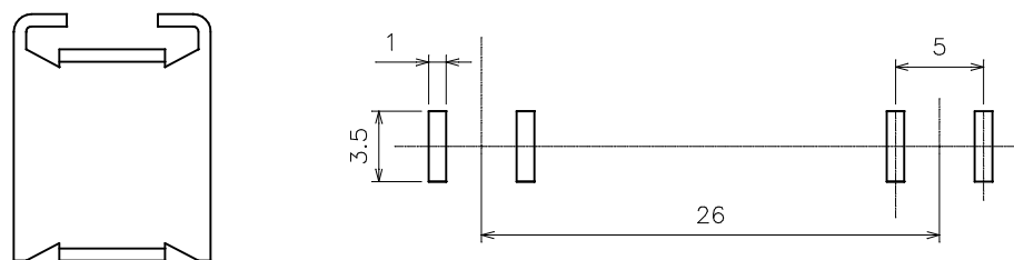
取付穴寸法参考図
