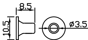
端子3.5φ
