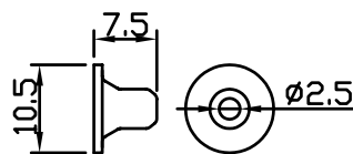
端子2.5φ
