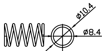
バネ
